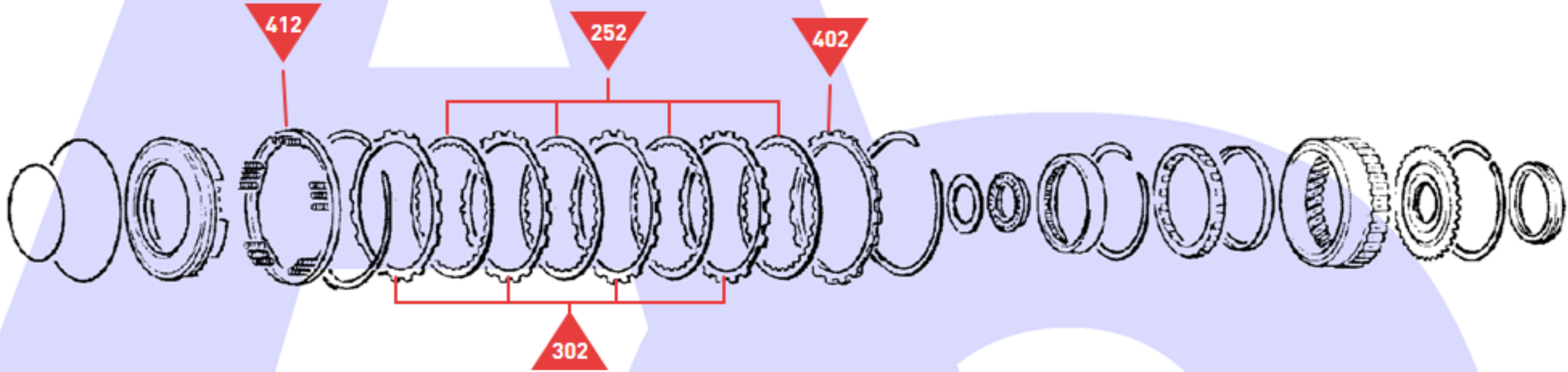
'B3' Brake & 'F2' Sprag
