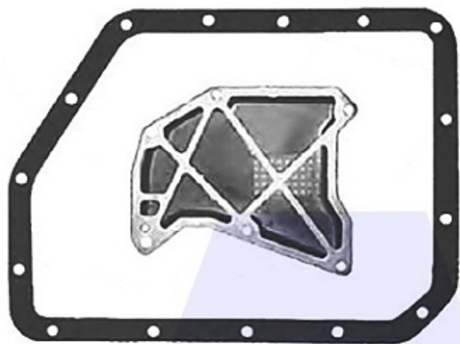
A210 Pan Gasket A210.GAS01 Filter A210.FIL01
