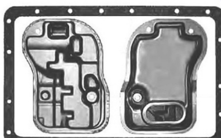
AISIN WARNER A341E LEXUS, VOLVO Pan Gasket A340.GAS01 Filter A341E.FIL02 1994-ON
