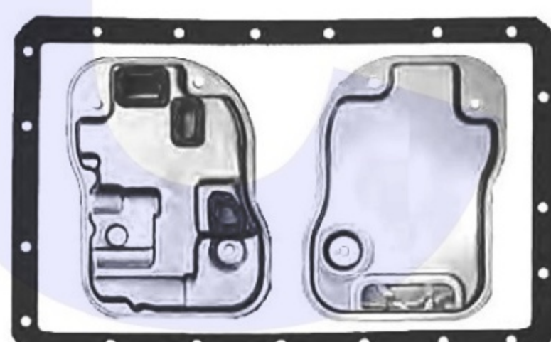
AISIN WARNER A350E Pan Gasket A340.GAS01 Filter A350.FIL01 1996-1998
