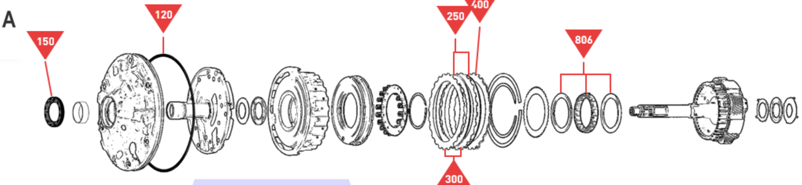
O. D. Direct Clutch
