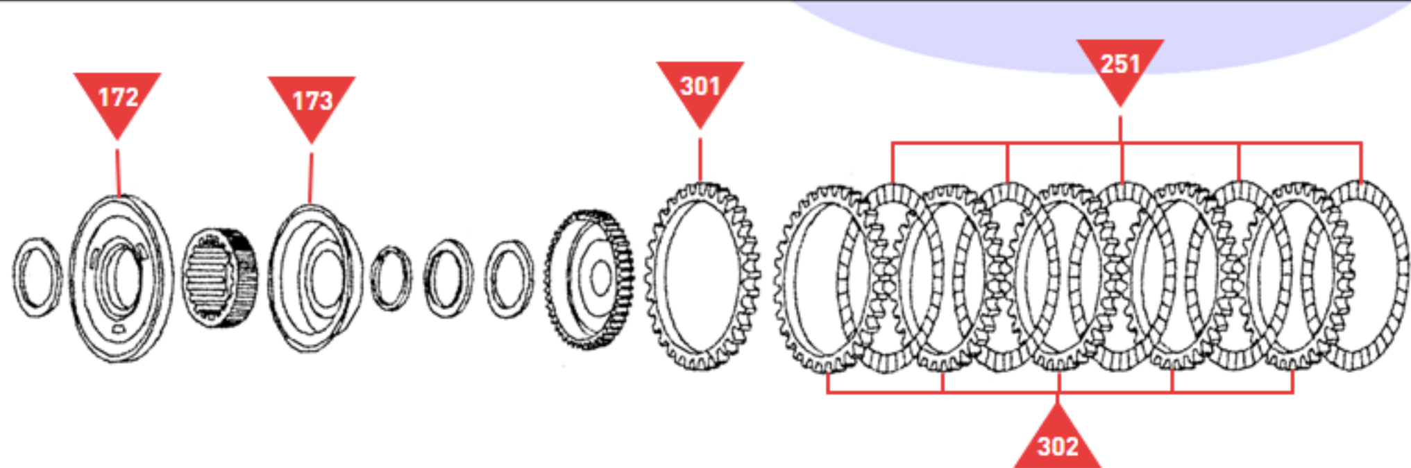
'C2' Clutch
