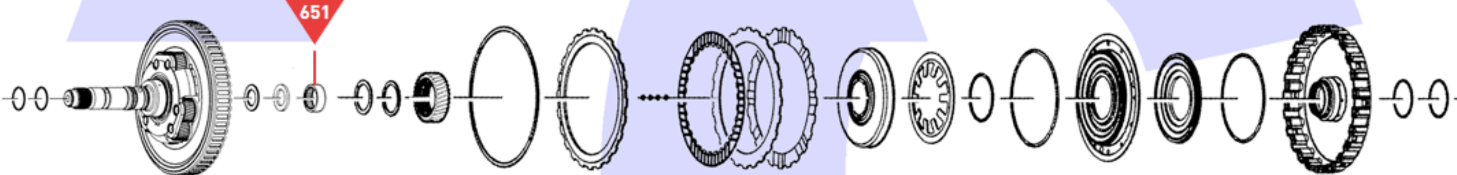
Input Shaft
