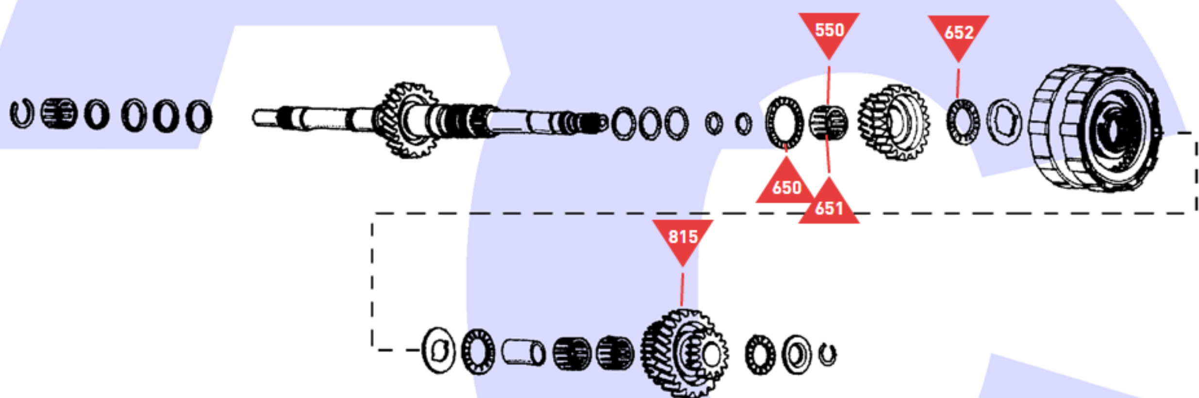
Mainshaft
