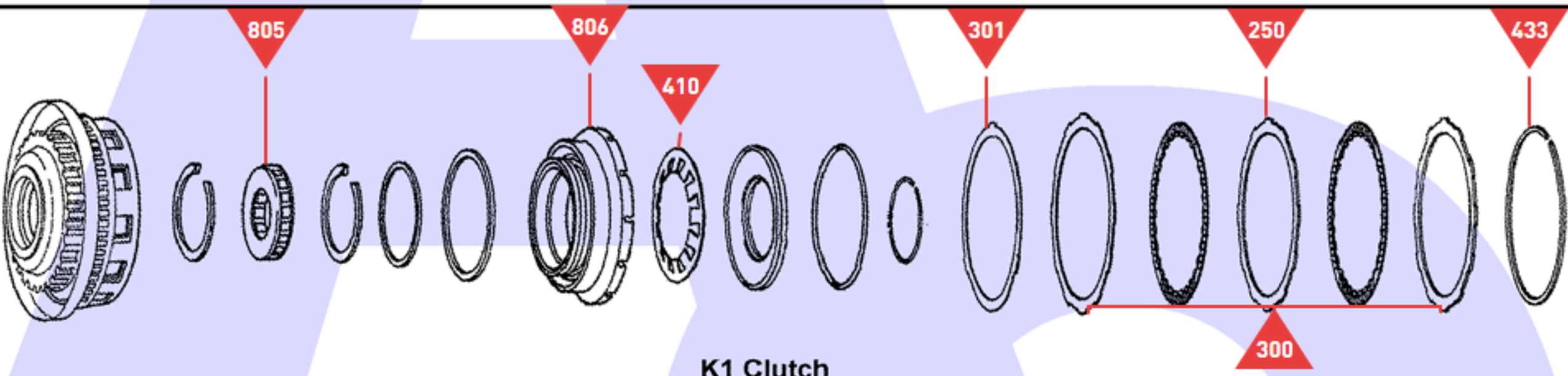
K1 Clutch
