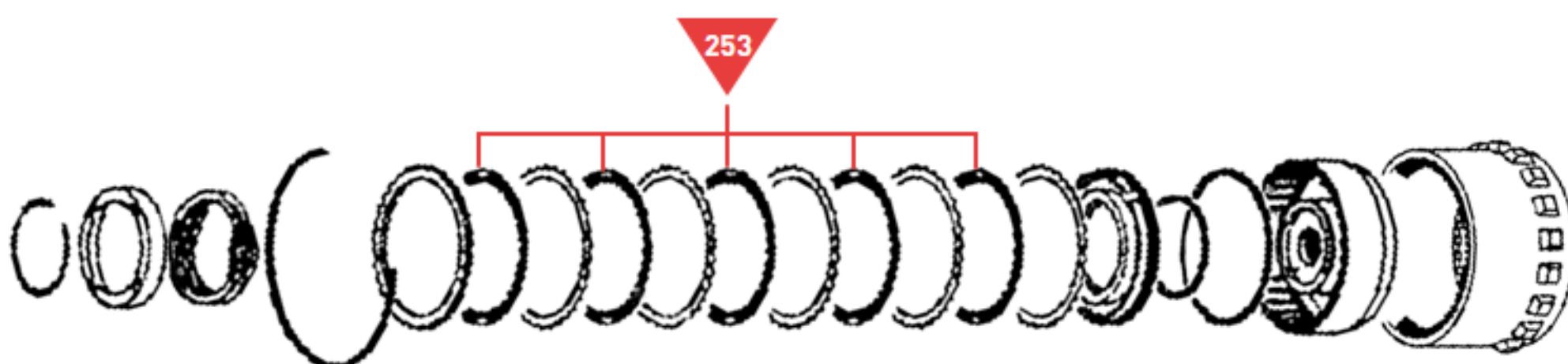
End (Overdrive) Clutch
