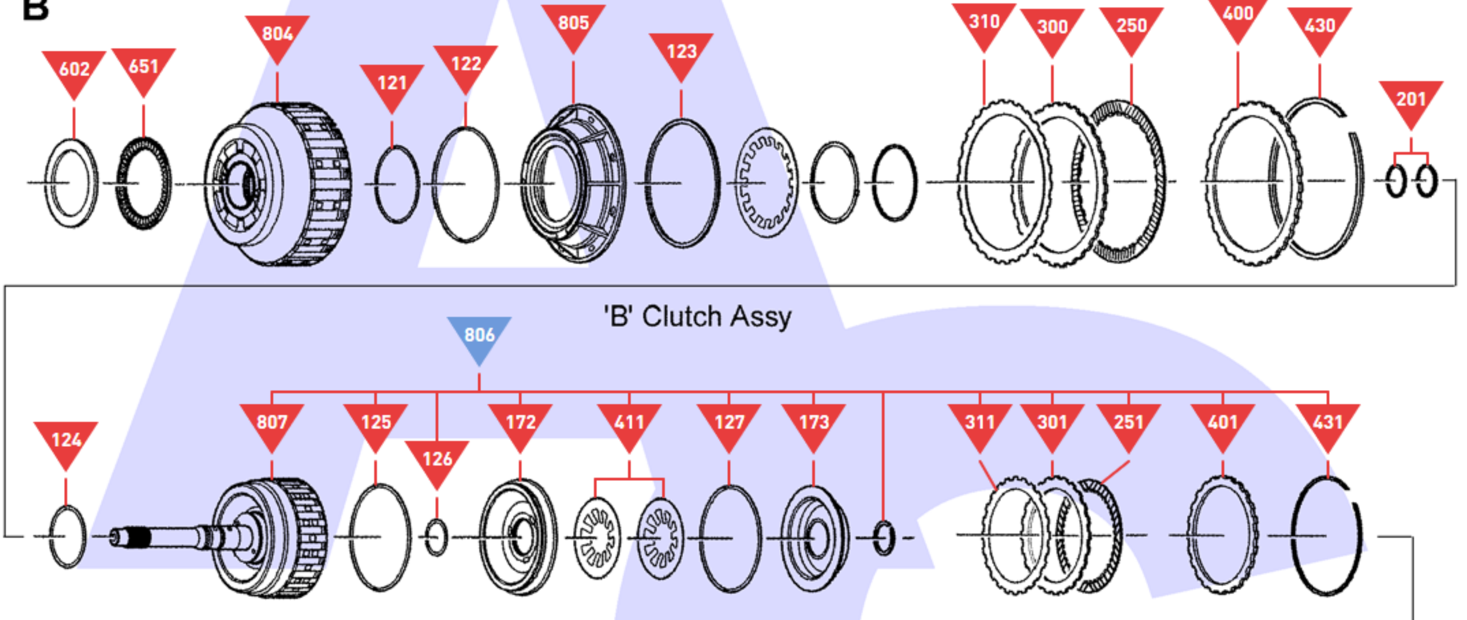
'B' Clutch Assy
