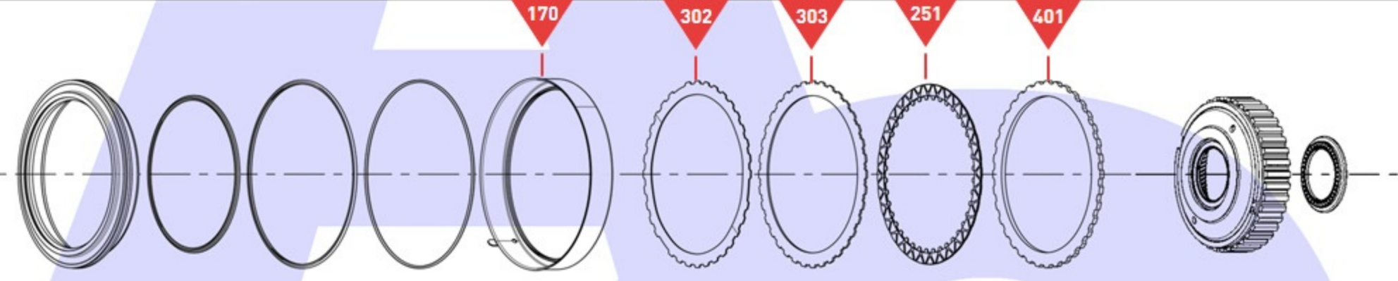
'B' Clutch
